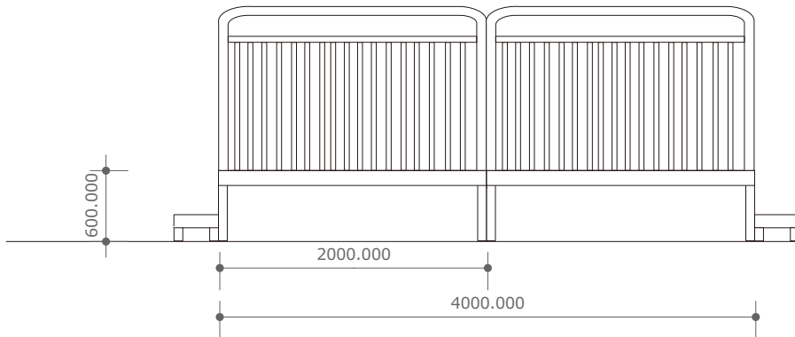
正面図
