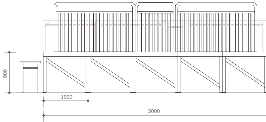
正面図
